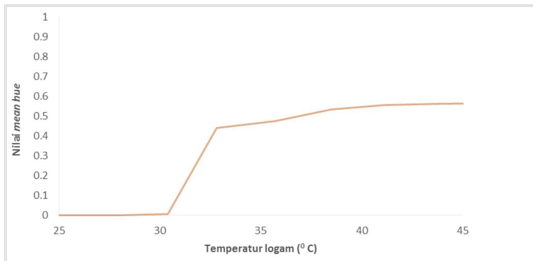
Gambar 7. (color online) Grafik hubungan nilai mean hue permukaan TLC terhadap kenaikan temperatur logam
