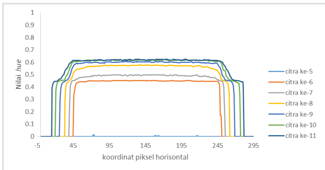
Gambar 8. ( color online ) Distribusi nilai hue sepanjang garis tengah citra permukaan TLC yang mengalami kontak dengan permukaan logam kuningan
