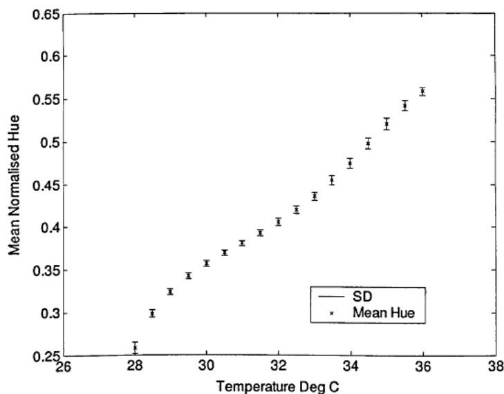
Gambar 1. Grafik hubungan antara nilai hue citra permukaan TLC dengan temperatur plat logam [3]
