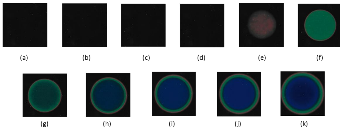
Gambar 5. (color online) Citra RGB permukaan TLC saat kontak dengan permukaan logam kuningan, pada detik ke (a) 0 (b) 30 (c) 60 (d) 90 (e) 120 (f) 150 (g) 180 (h) 210 (i) 240 (j) 270 (k) 300
