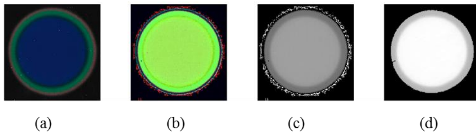
Gambar 6. (color online) Hasil pengolahan citra permukaan TLC saat kontak dengan permukaan logam kuningan, pada detik ke 270, (a) citra RGB (b) citra HSV (c) citra komponen hue (d) citra akhir
