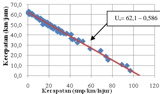
Gambar 6. Hubungan kecepatan dan kerapatan pada ruas jalan Bandung-Nagreg
