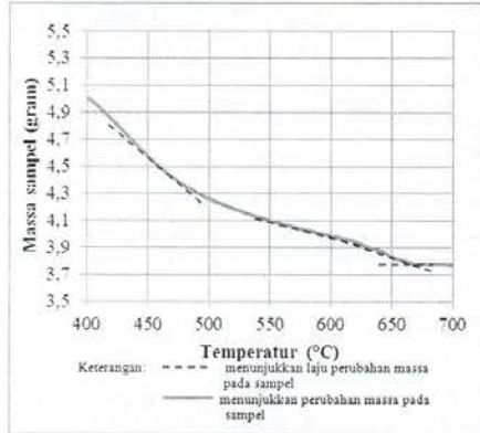
Gambar 3. Kurva hasil TGA blotong
