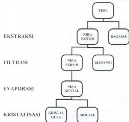
Gambar 1. Bagan proses pembuatan gula
