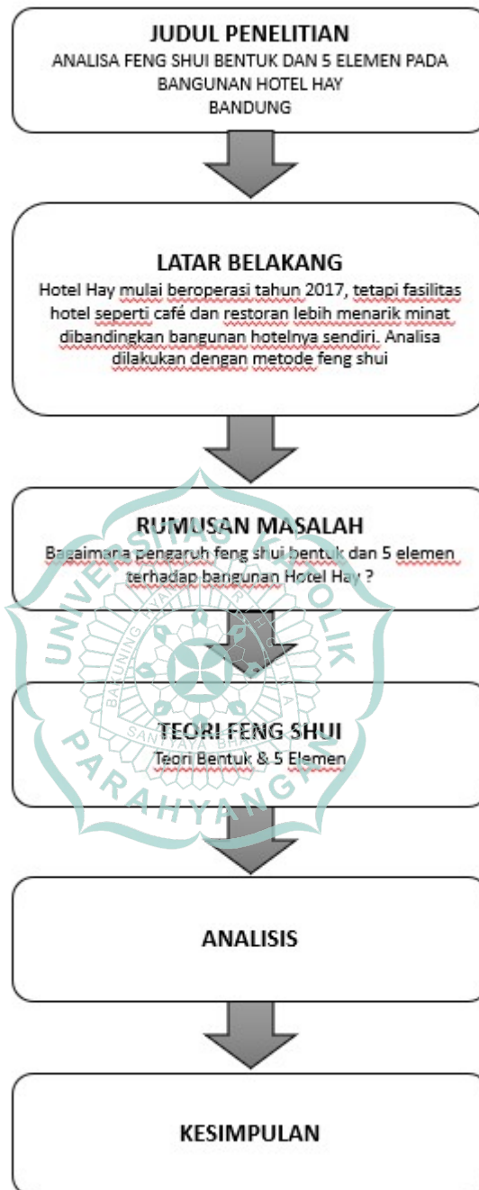
Gambar 1.3 Kerangka Penelitian
